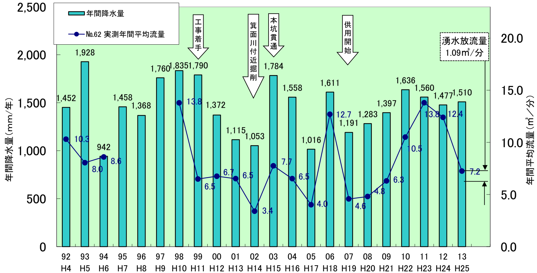
箕面大滝付近 年間降水量と年間平均流量(実測)の関係
