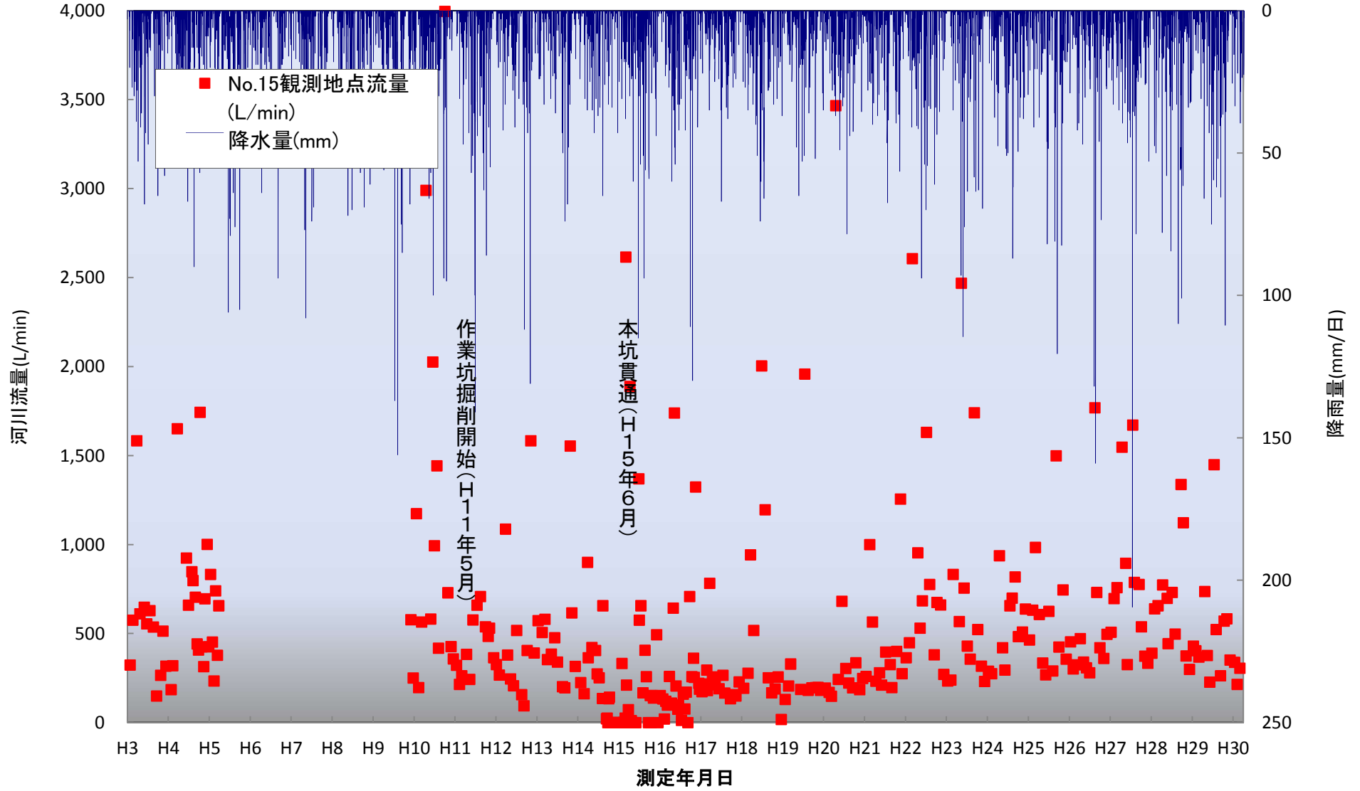
箕面有料道路 河川流量観測結果(No.15: 茶長阪川)
