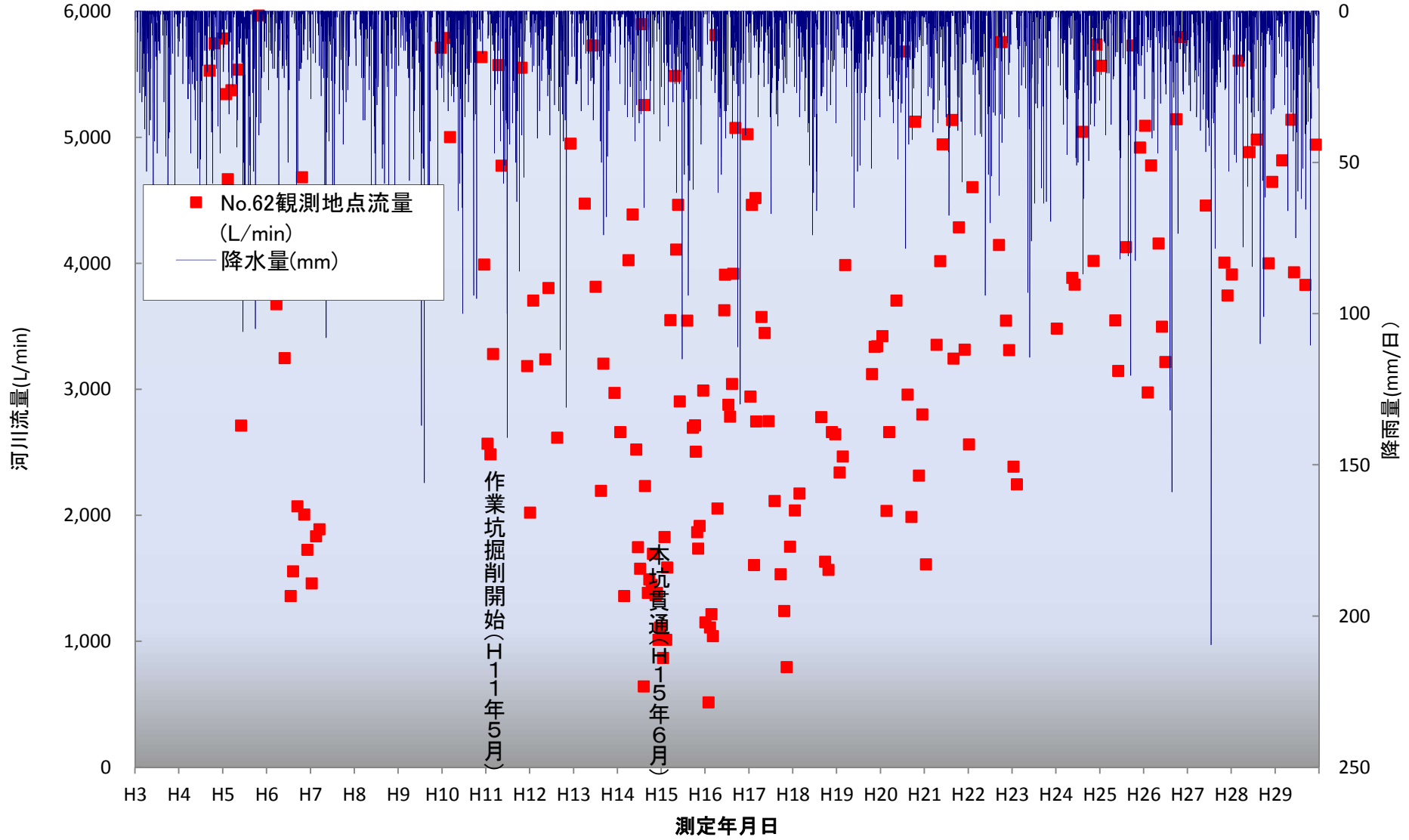
箕面有料道路 河川流量観測結果(No.62: 箕面川)
