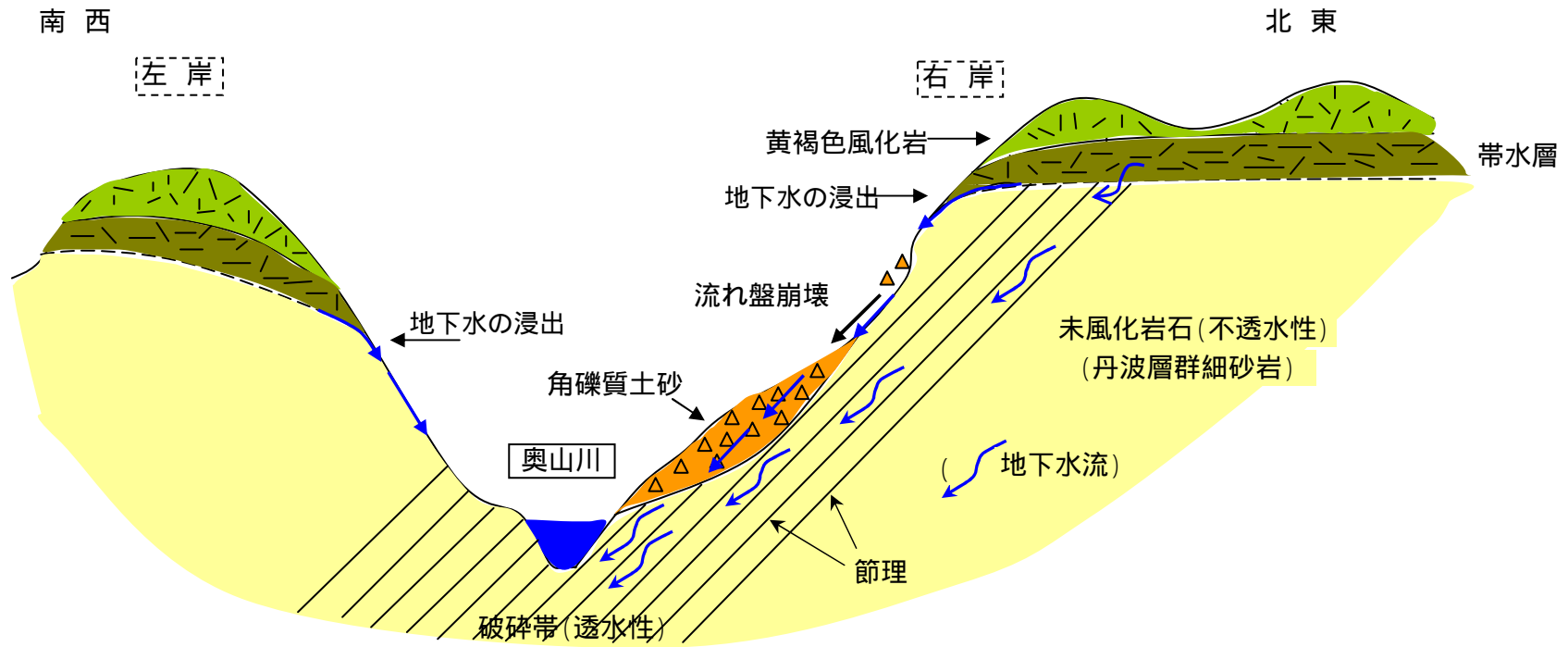
図-7 斜面崩壊 イメージ図
