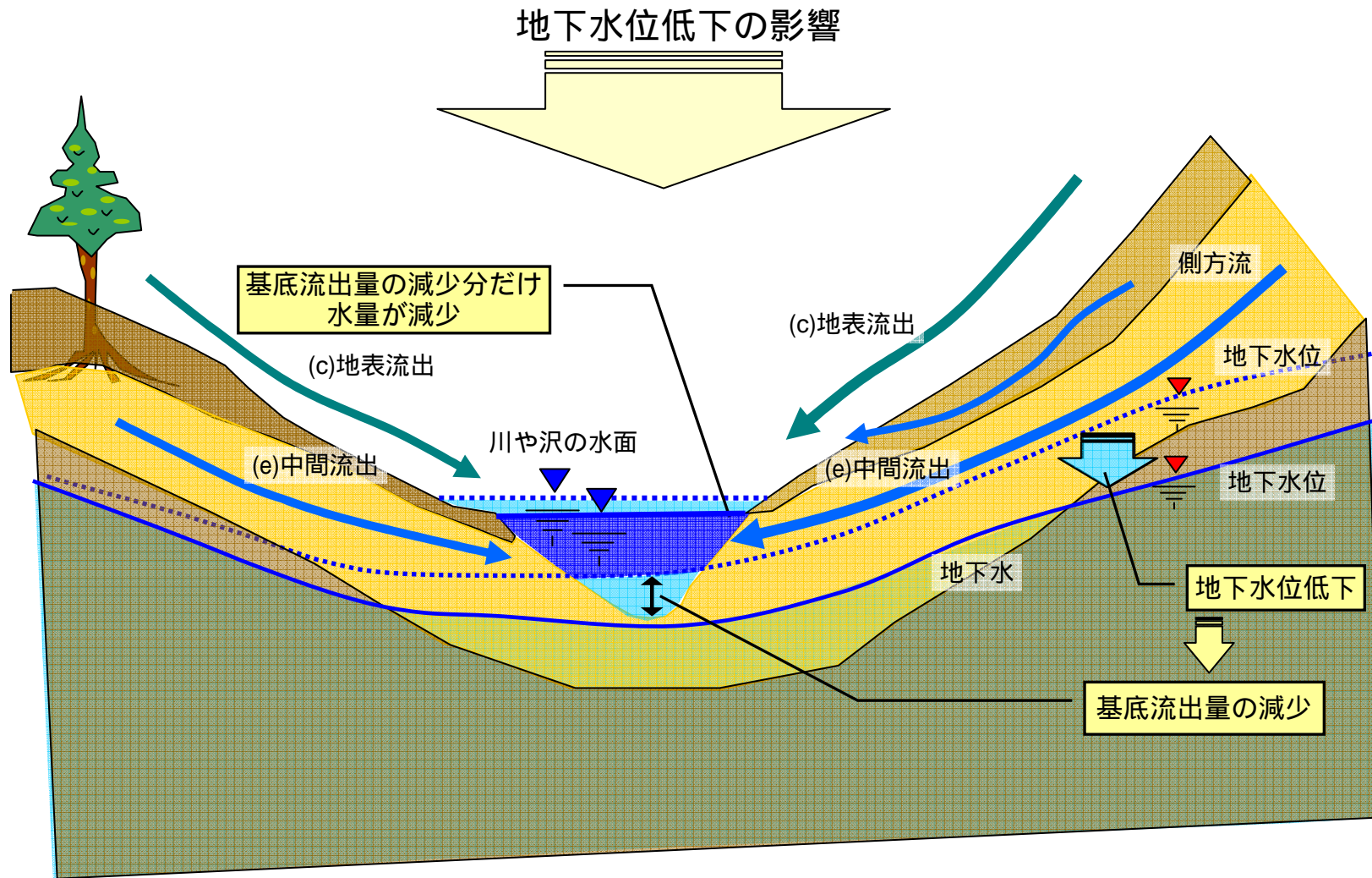
図 - 5 - 2 地下水位低下の影響 イメージ図
